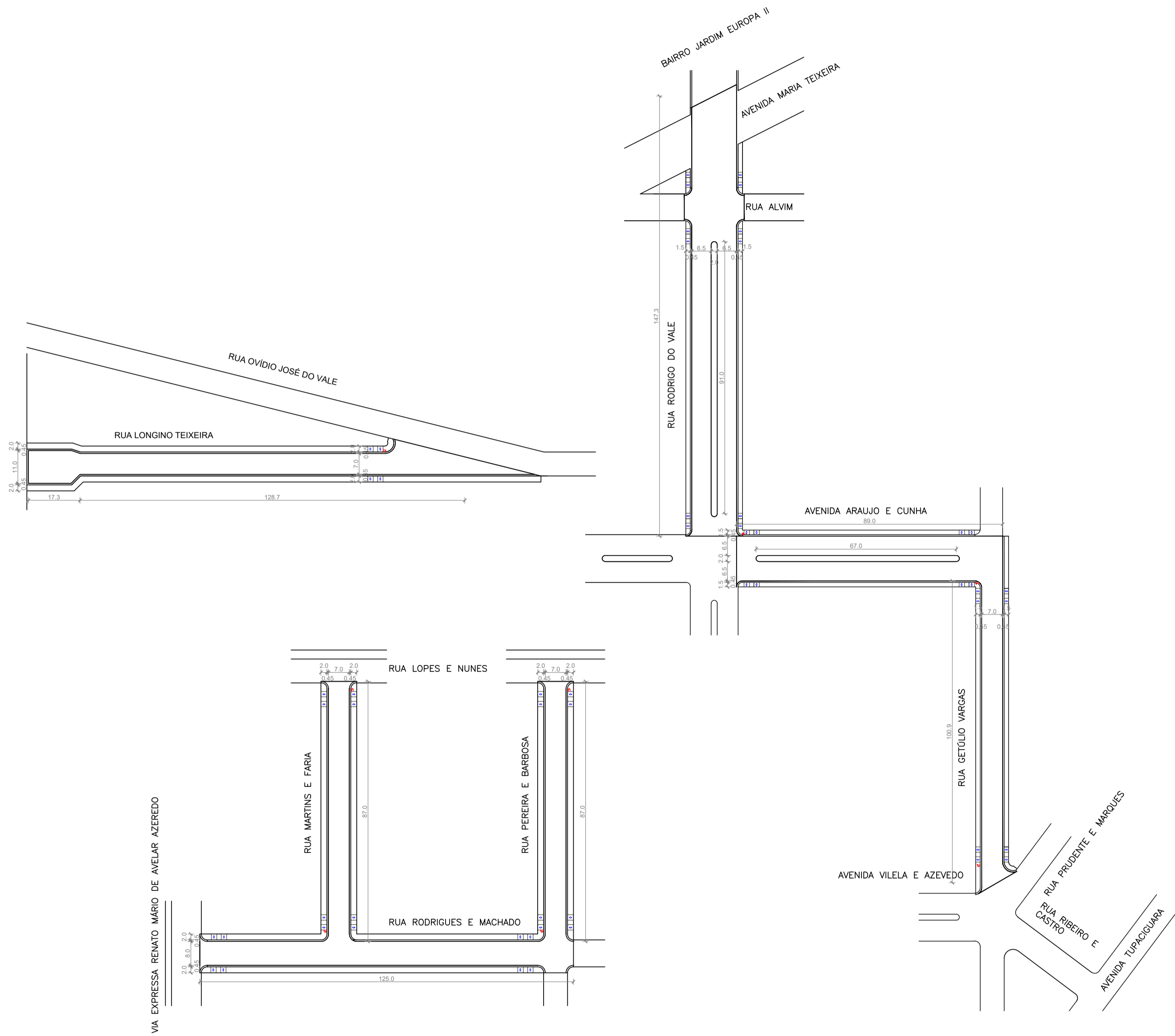
PLANTA BAIXA ESC: 1/1000
