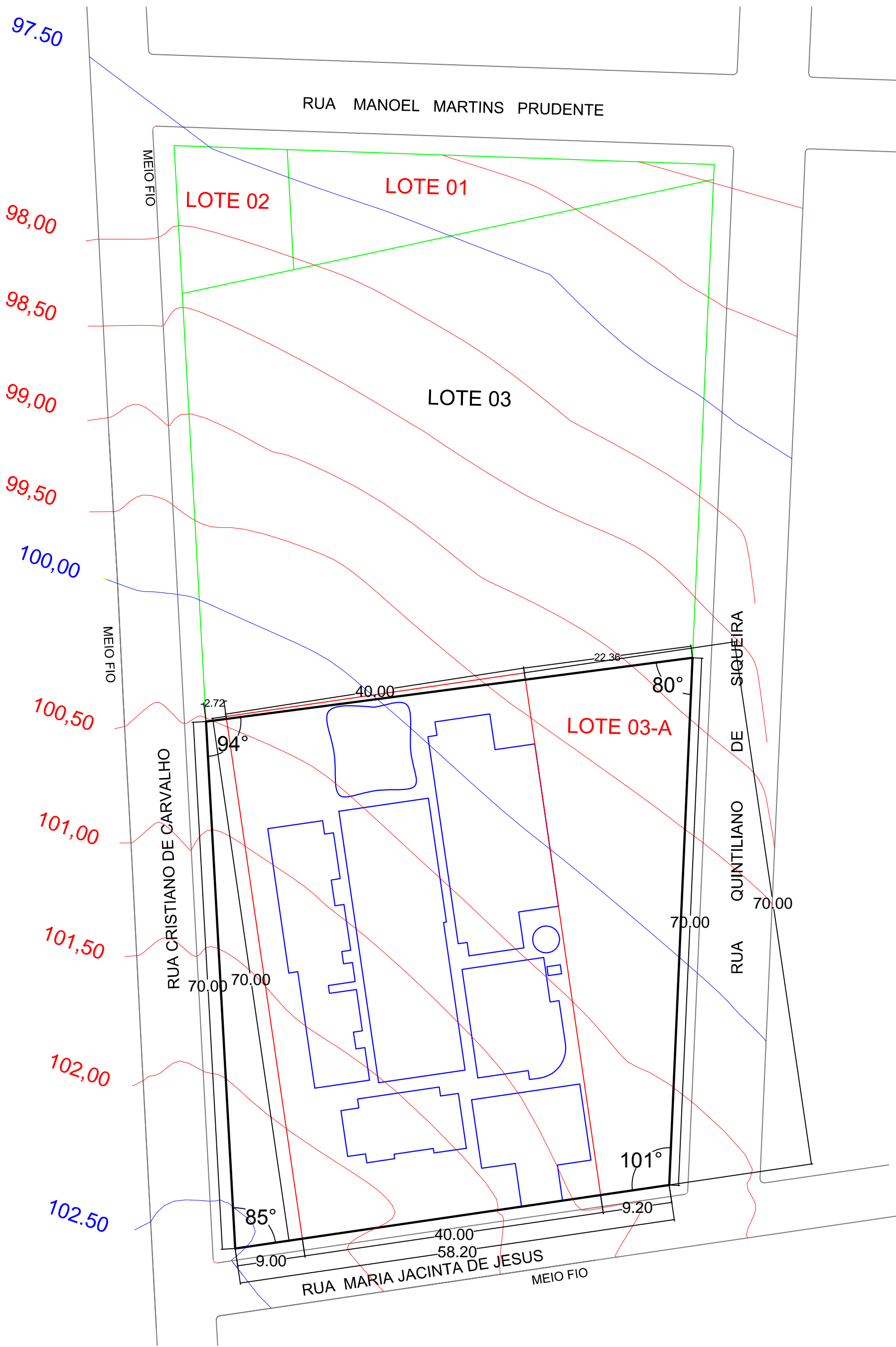
PLANTA DE LOCAÇÃO DA CRECHE PRO-INFÂNCIA TIPO B escala 1/500 Rua Maria Jacinta de Jesus - Qd Lt 03-A Bairro Morada Nova - TUPACIGUARA-MG
